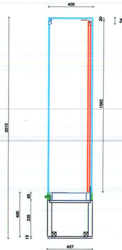
Seitenansicht
