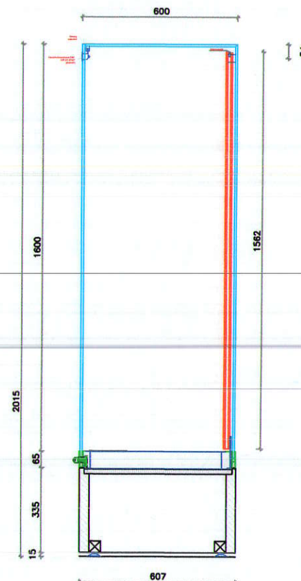
Seitenansicht
