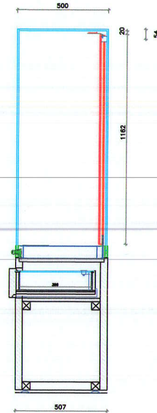
Seitenansicht
